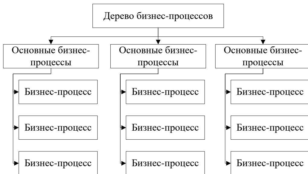
1 – Модель бизнес-процессов
