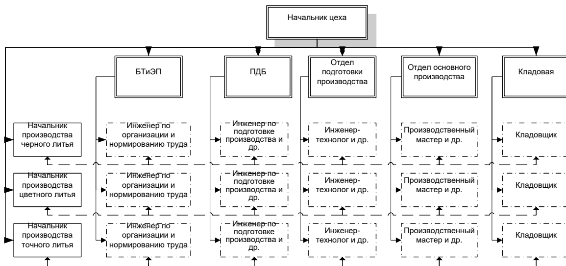
Рисунок 2 – Матричная модель
